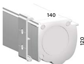
Sujeción a pared (en mm.)
