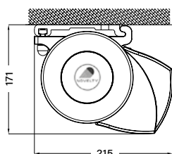
Instalación en el techo (en mm.)
