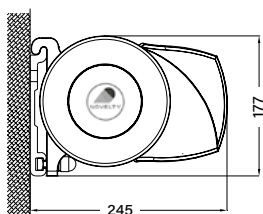
Instalación en la pared (en mm.)
