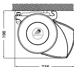
Instalación en el techo (en mm.) Para colocación a techo es imprescindible el uso de soportes especiales.
