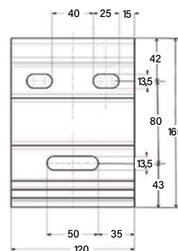
Placa de sustentación (en mm.)
